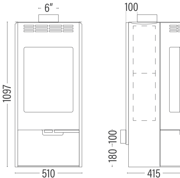
Optional Heatbank
