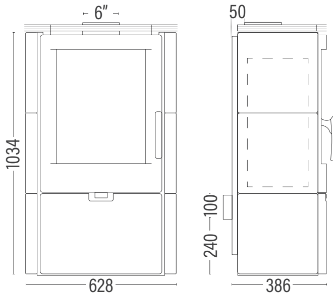
Optional Heatbank
